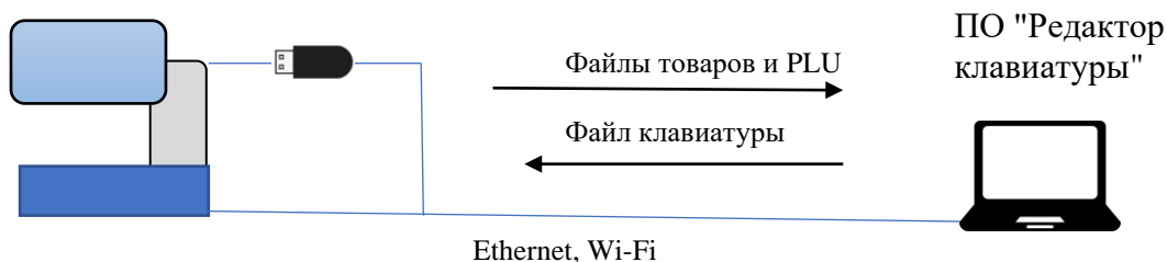
Рис. 6. Схема формирования персональной клавиатуры
