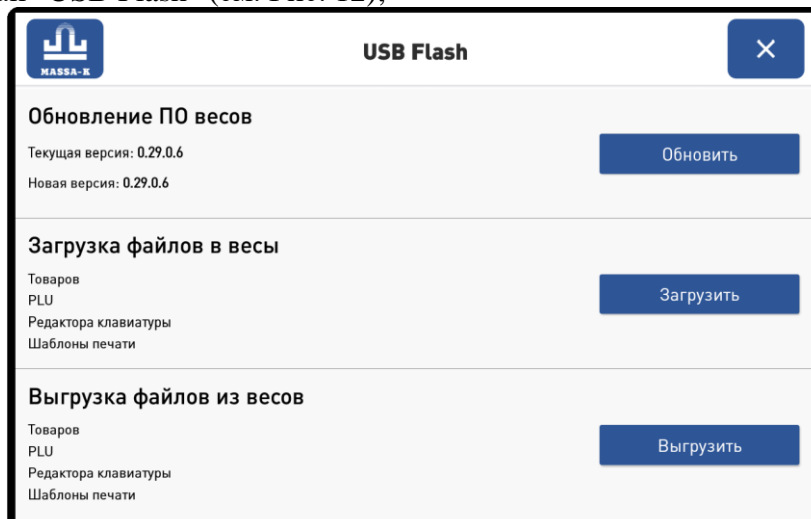
Рис. 12. Экран "USB Flash"
