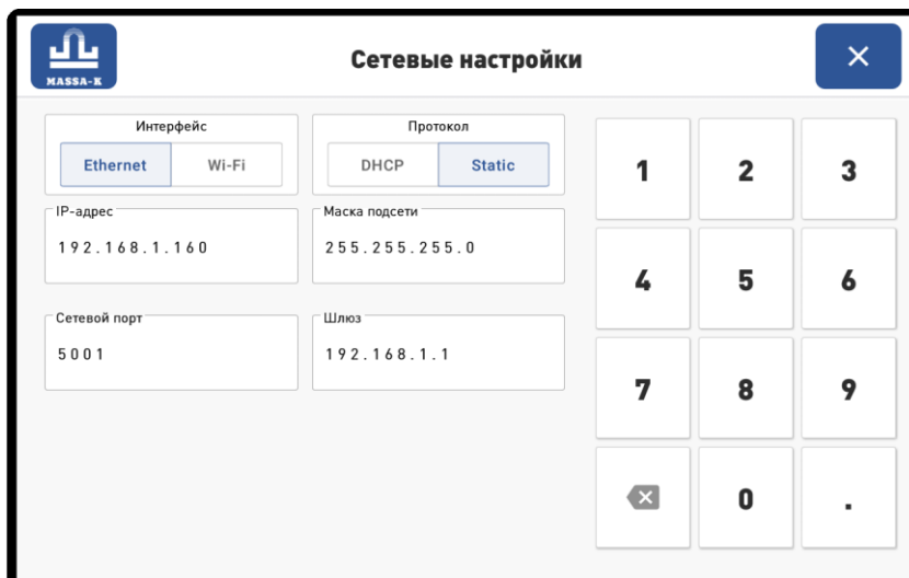
Рис. 13. Экран "Сетевые настройки"
